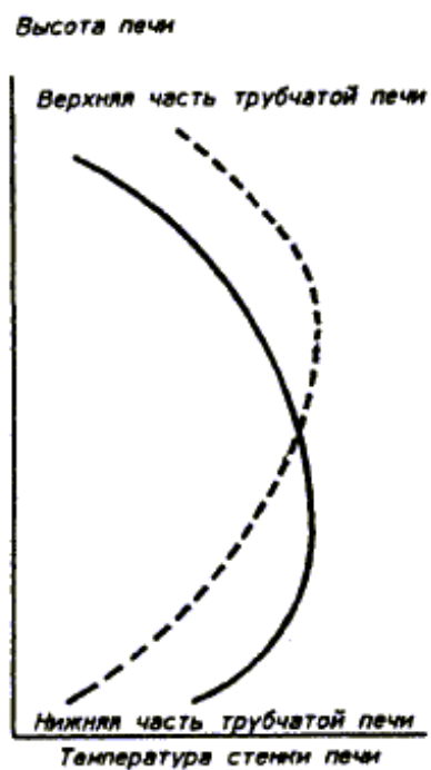
Рис. А8. Температурные профили стенки печи
