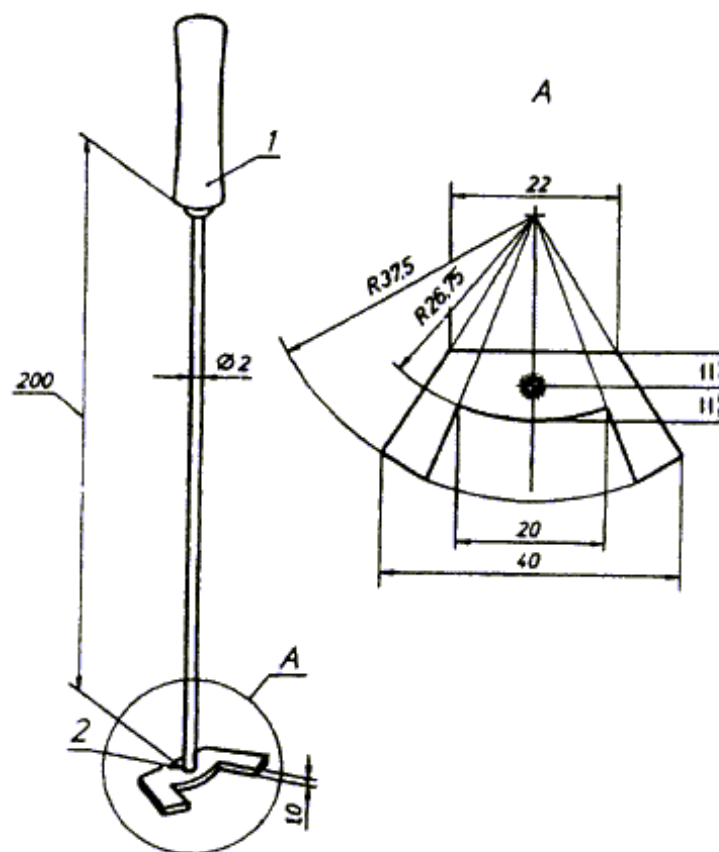
1 — деревянная ручка; 2 — сварной шов
