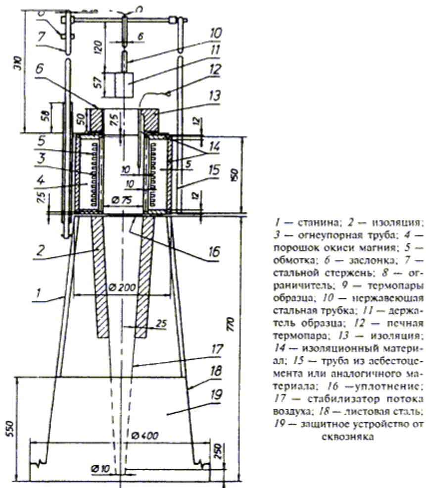
Рис. А1. Общий вид установки
